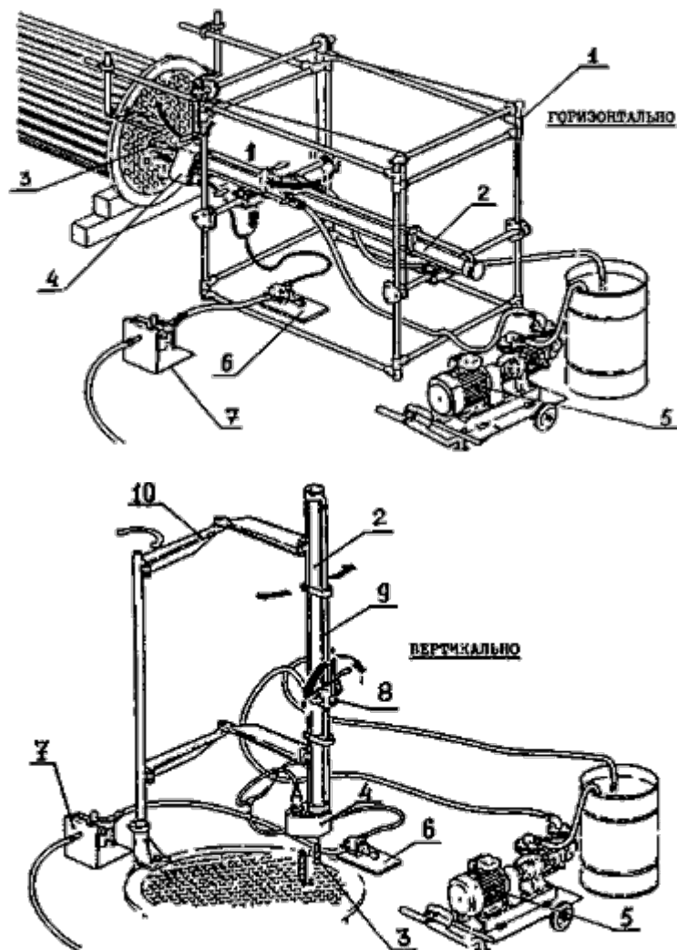
Рисунок 8 - Общий вид установки "Трубоочиститель-2000"
