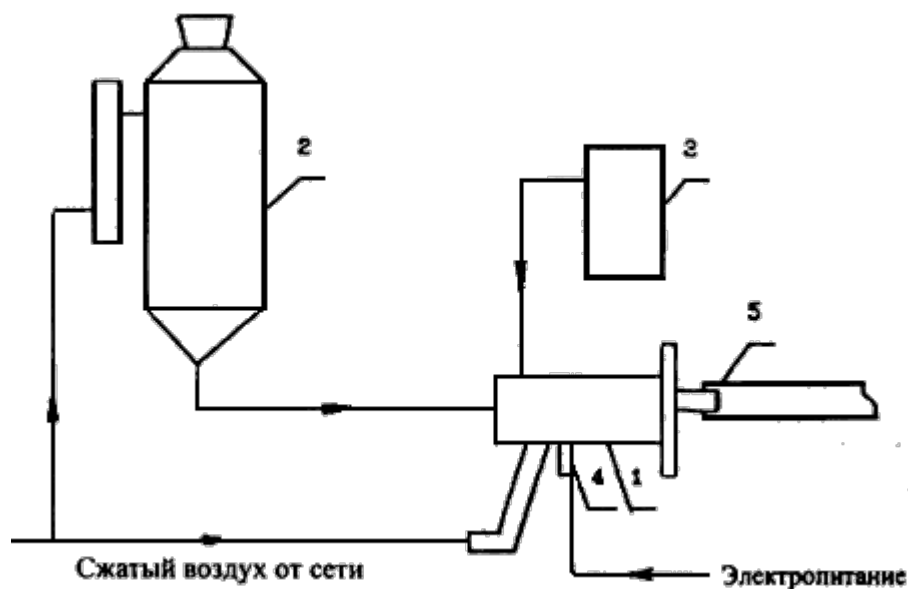
Рисунок 1 - Принципиальная схема очистки трубок термоабразивным способом
