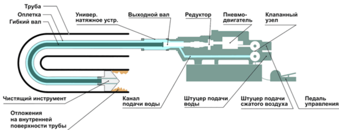
Рисунок 3 - Установка "Крот"
