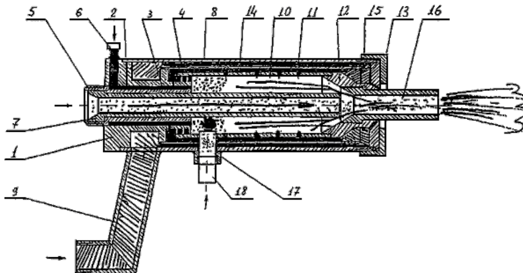
Рисунок 2 - Устройство для струйно-абразивной очистки
